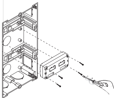
Pulsadores del 81 al 96 Push-buttons 81 to 96 Poussoirs de 81 à 96
