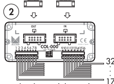
Pulsadores del 17 al 32 Push-buttons 17 to 32 Poussoirs de 17 à 32
