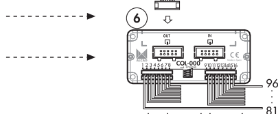
Pulsadores del 81 al 96 Push-buttons 81 to 96 Poussoirs de 81 à 96
